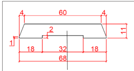
Zachthout voorgeverfd trapezium
